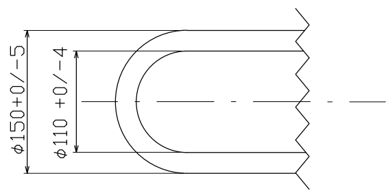
SECTION 'A-A' (エレメント本体部)
